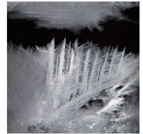
結晶の例
